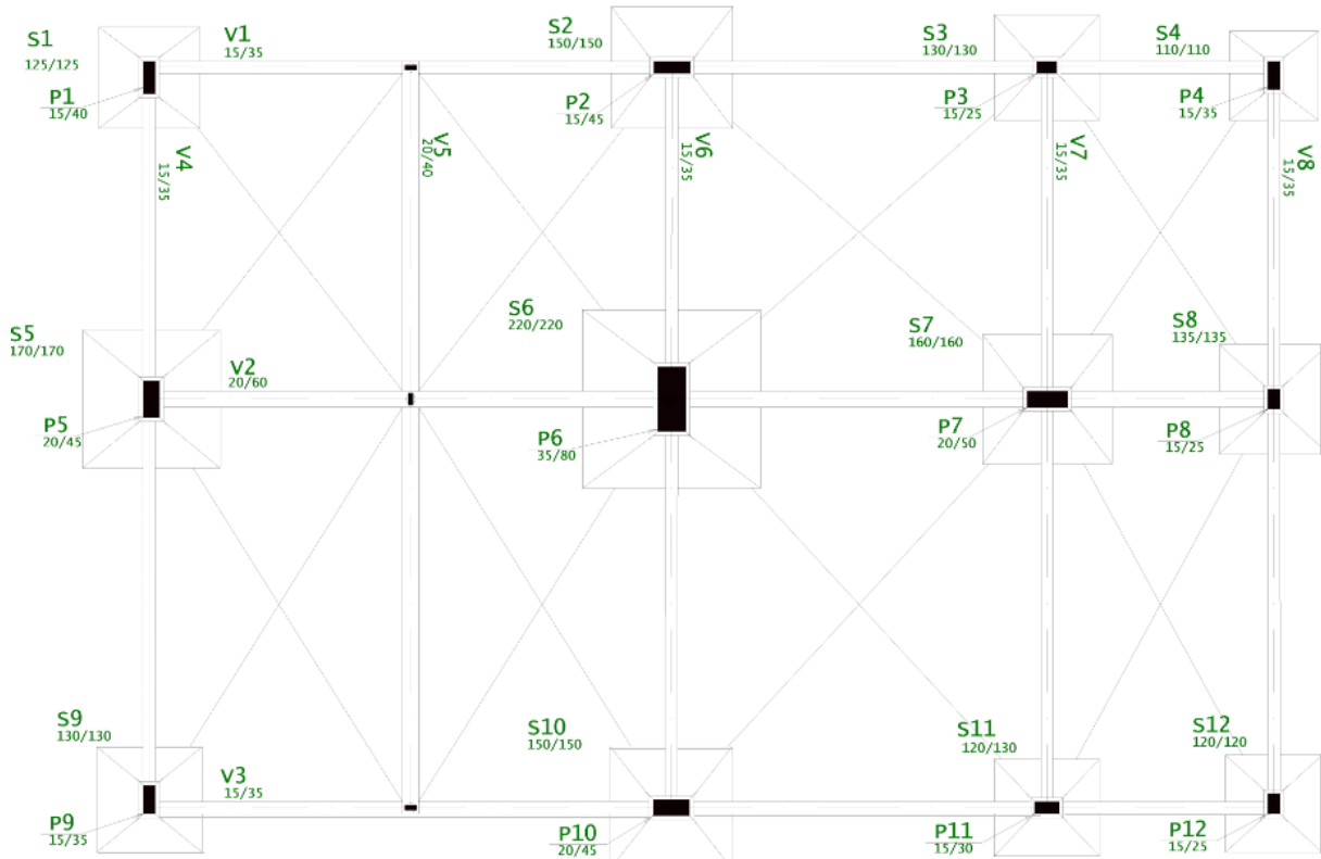
FIGURA 6 – Planta de fundação referente ao projeto estrutural Proj.3
