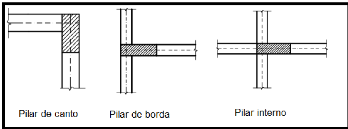
FIGURA 1 - Classificação dos pilares quanto à posição
