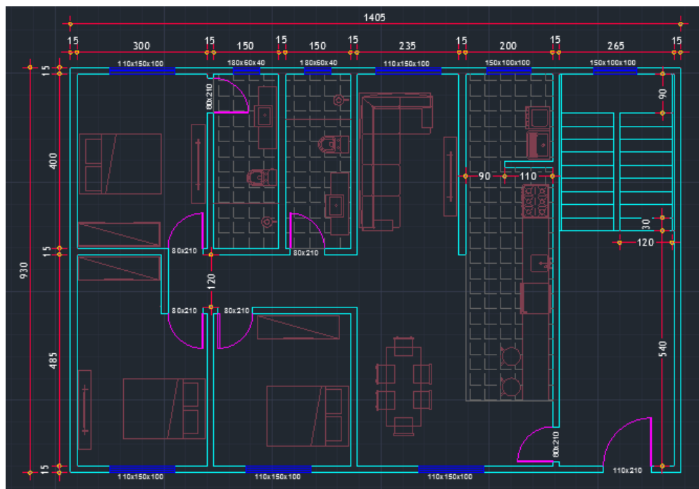
FIGURA 3 - Projeto arquitetônico
