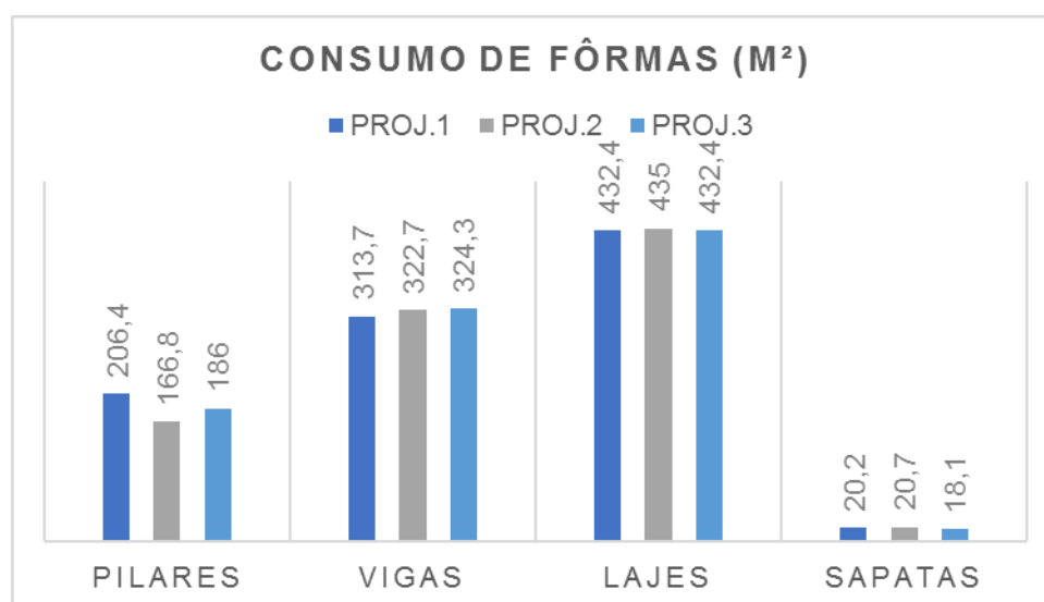
GRÁFICO 1- Gráfico referente a quantidade de fôrmas (m 2 ).
