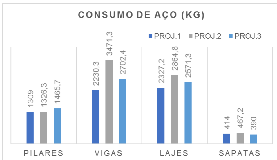
GRÁFICO 2- Gráfico referente a quantidade de aço (kg)
