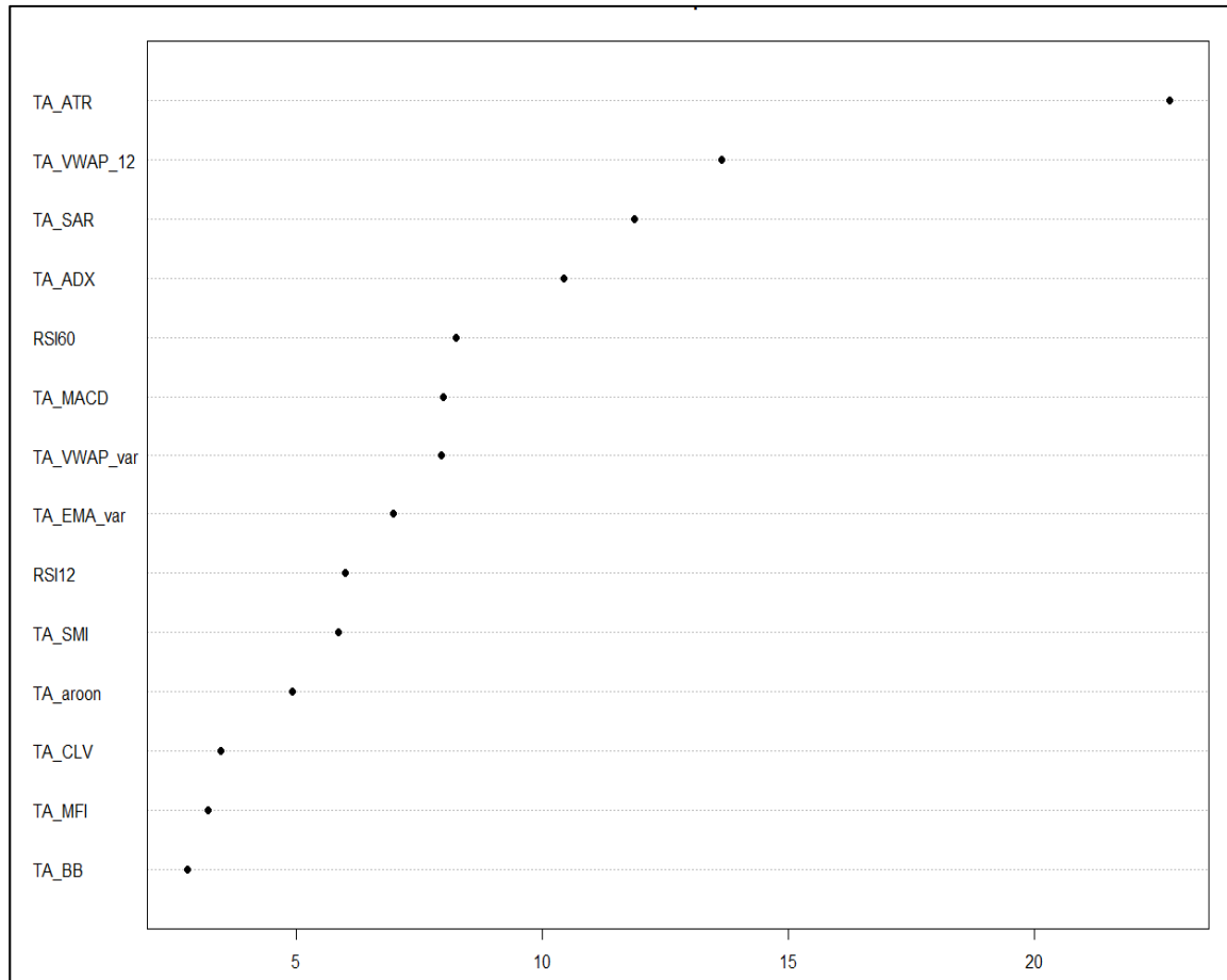
Figure A III.1 Importance des variables en utilisant un modèle de forêts aléatoire
