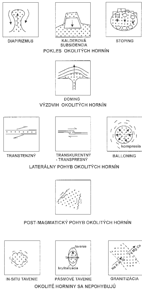
Obr. 1. Spôsob výstupu a umiestnenia granitoidných telies v kôre (prevzaté z Clarke, 1992).
