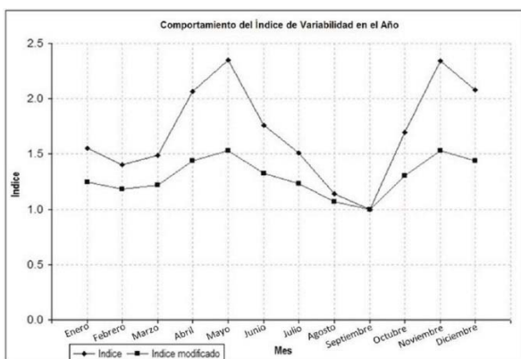
Fig. 2. Índice obtenido a partir del caudal medio multianual Estación Limnigráfica Mateguadua - Periodo: 1975-1995.
