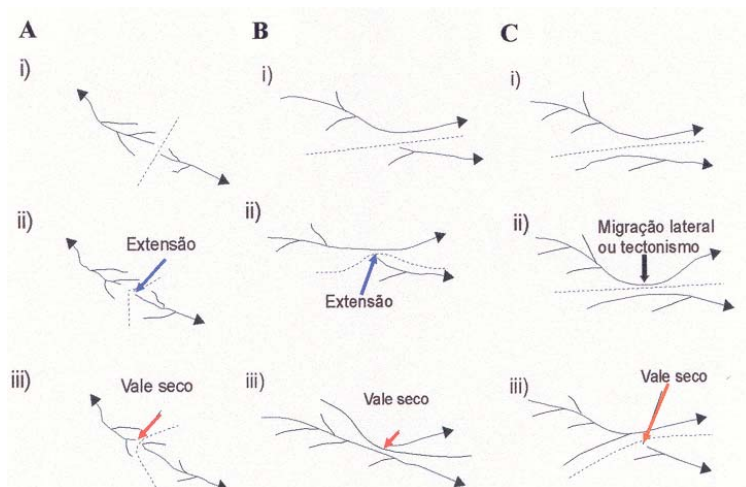
Figura 3 Formas de rearranjo de drenagem através de captura vistas em planta. A linha tracejada é o divisor da drenagem. (A) capturas por extensão da cabeceira, (B) e (C) capturas através de invasão lateral de uma bacia de drenagem adjacente, ou através de extensão de cabeceira de um tributário (B) ou migração lateral de um rio para capturar um tributário adjacente (C). Em todas as situações espera-se rejuvenescimento de cabeceira do rio capturado no ponto de captura ou a montante deste. Modificado de Bishop (1995).
