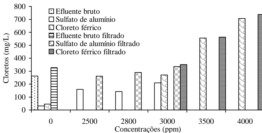
FIGURA 5: Caracterização dos valores de cloretos (mg/L) do efluente bruto não filtrado e filtrado, submetidos aos tratamentos com sulfato de alumínio e cloreto férrico, ambos não filtrado e filtrado.
