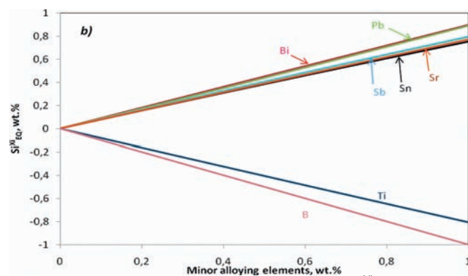
Figure 3 b - The effect of minor alloying elements on the Si_{EQ}^{Xi} for hypoeutectic alloys. Slika 3 b - Uticaj minornih legirajućih elemenata na Si_{EQ}^{Xi} za hipotetičke legure
