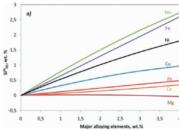
Figure 3 a - The effect of major alloying elements on the Si_{EQ}^{Xi} for hypoeutectic alloys Slika 3 a - Uticaj glavnih legirajućih elemenata na Si_{EQ}^{Xi} za hipotetičke legure
