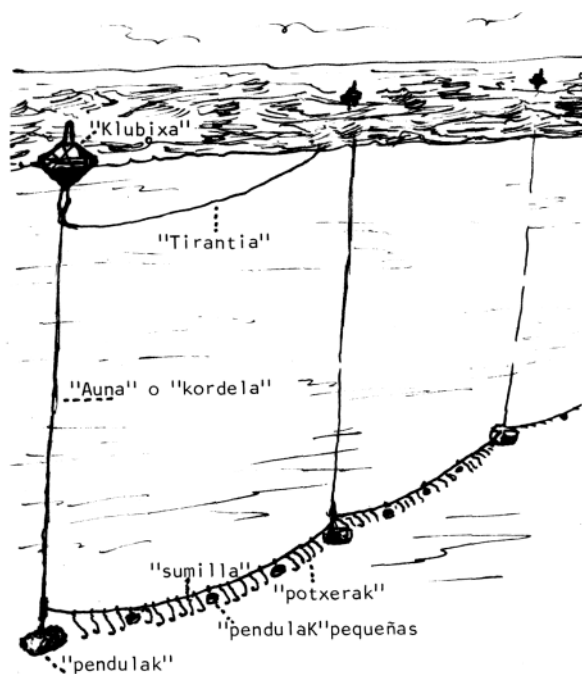
Fig. 2.— Palangre besugero
