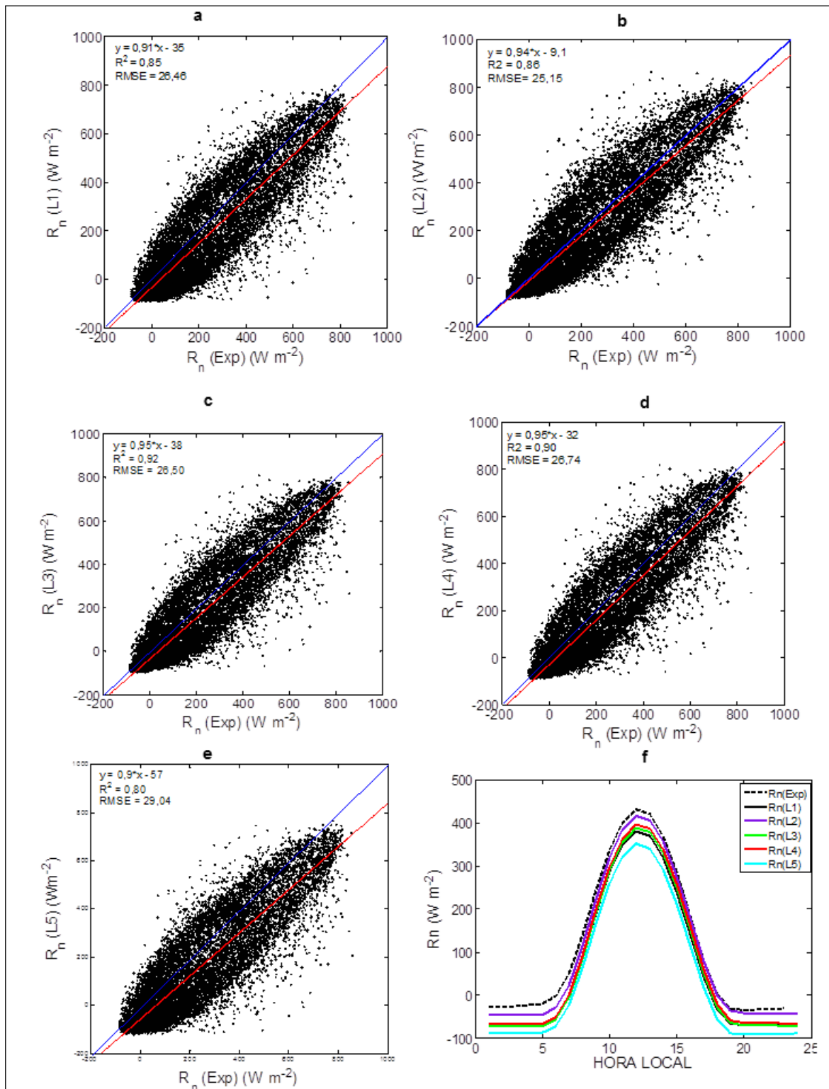
Figura 1- Dispersão entre dados experimentais e simulados com diferentes equações de radiação de onda longa incidente pelo modelo SiB2 no bioma Pampa: figura 1 (a) L1; figura 1 (b) L2; figura 1 (c) L3; figura 1 (d) L4; figura 1 (e) L5 e figura 1 (f) ciclo diário médio do saldo de radiação. Linhas coloridas contínuas representam os resultados simulados pelo modelo SiB2 e a linha tracejada preta representa os dados experimentais.
