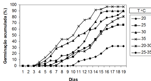
FIGURA 1: Porcentagem média de germinação acumulada de sementes Jatobá-Mirim em seis temperaturas.
