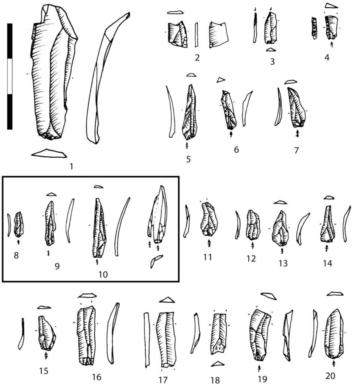
Fig. 9. Útiles retocados y soportes laminares del nivel IXb: 1: Lámina; 2-3 Laminilla de dorso marginal con huellas de impacto; 4 Laminilla de dorso; 5-14 Laminillas provenientes de núcleo tipo raspador carenado (8-10 remontan); 15-20 laminillas provenientes de núcleos prismáticos.
