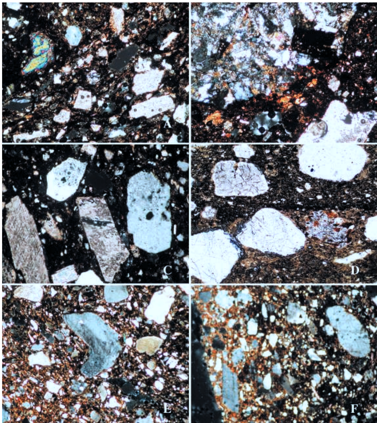
Plancha 6. Microfotografías mostrando diversos aspectos petrográficos de cerámicas. 6A: Pasta con piroxenos y como desgrasantes añadido carbonatos en una muestra del Castro de Peñas de Oro (Vitoriano, Álava), 6B: (Mismo yacimiento) Cerámica con fragmentos de subofitas y como desgrasante añadido carbonatos. 6C: (Mismo yacimiento) Cerámica con Jacintos de Compostela y como desgrasante añadido carbonatos. 6D: Granos de arena muy redondeados en una cerámica de época romana (Oiasso, Irún, Guipúzcoa). 6E: Feldespato con geometría redondeada adquirida durante el ciclo sedimentario y con geometría en forma de "L" posiblemente provocada por la trituration mecánica del barro (Ecce Homo, Alcala de Henares, Madrid). 6F: (Mismo yacimiento) feldespatos y cuarzoes muy redondeados junto con un fragmento de feldespato muy anguloso, posiblemente fracturado por acción mecánica del batido del barro.
