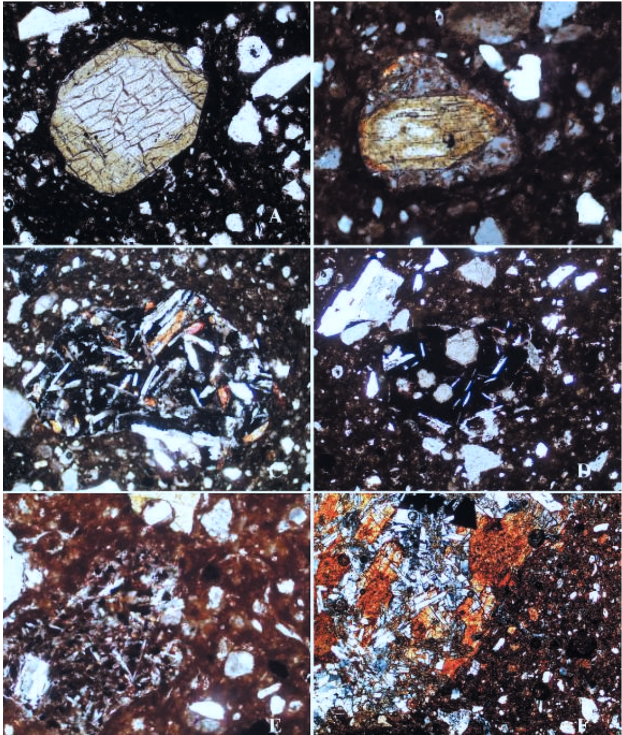
Plancha 3. Naturaleza de los diferentes tipos de desgrasantes ígneos. 3A y 3B : Piroxenos, en cerámicas del yacimiento de Moru (Elgoibar, Guipúzcoa), el segundo incluido en una plagioclasa 3C , 3D y 3E : (mismo yacimiento) fragmentos de rocas volcánicas de diferente naturaleza, mostrando vidrio volcánico y texturas ígneas. 3F : Fragmento de roca subvolcánica con textura ofítica en una cerámica procedente de Sansol (Muru Astrain, Navarra).
