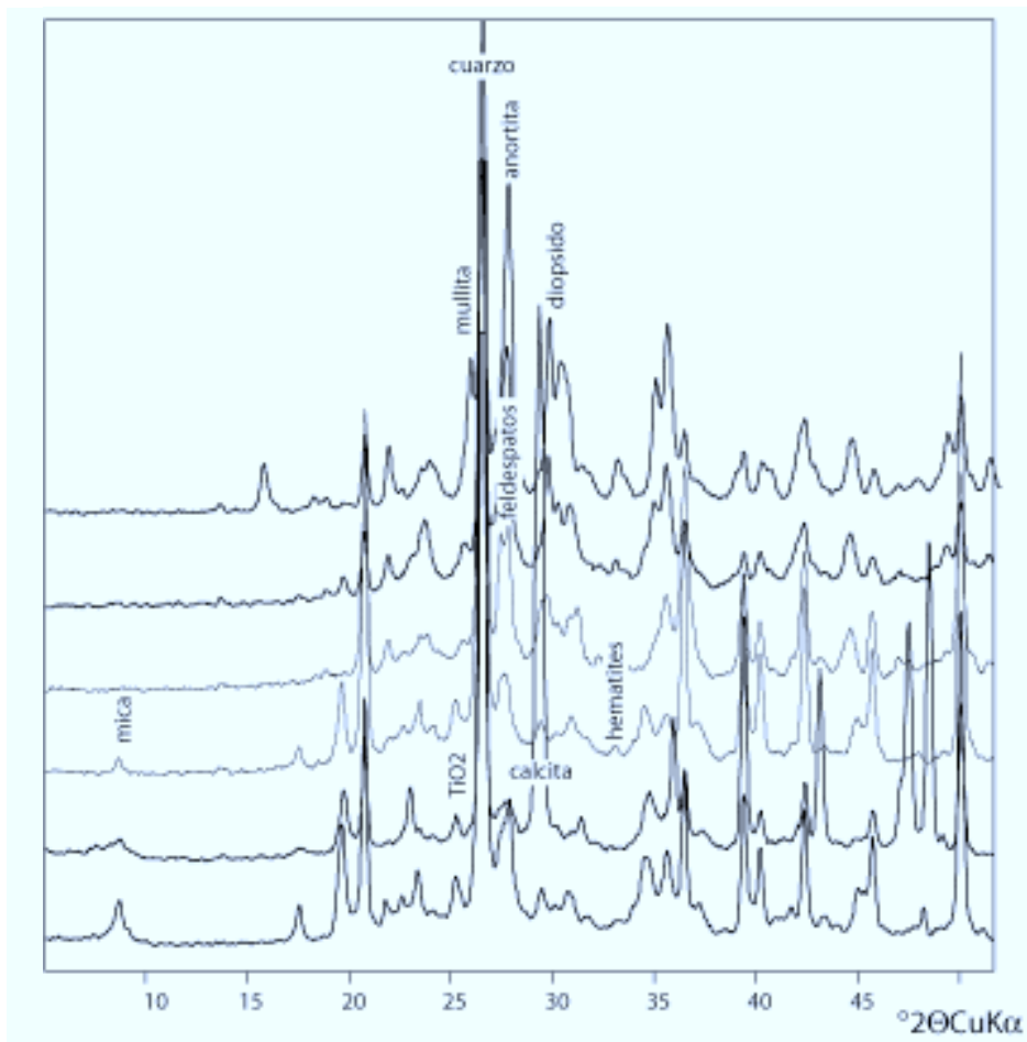
Figura 8. Difractogramas de cerámicas no carbonatadas vidriadas.
