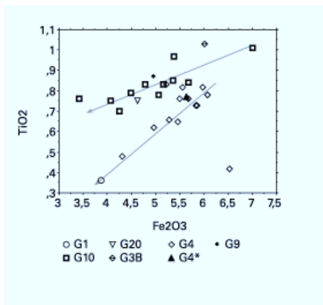
Figura 6: Diagrama de variación Fe 2 O 3 frente a TiO 2 en el que se incluyen otros grupos de cerámicas del mismo yacimiento de la Catedral de Santa María de Vitoria-Gasteiz (Álava). Obsérvese como los nuevos grupos de cerámicas se integran en las tendencias de variación marcadas por los grupos principales.
