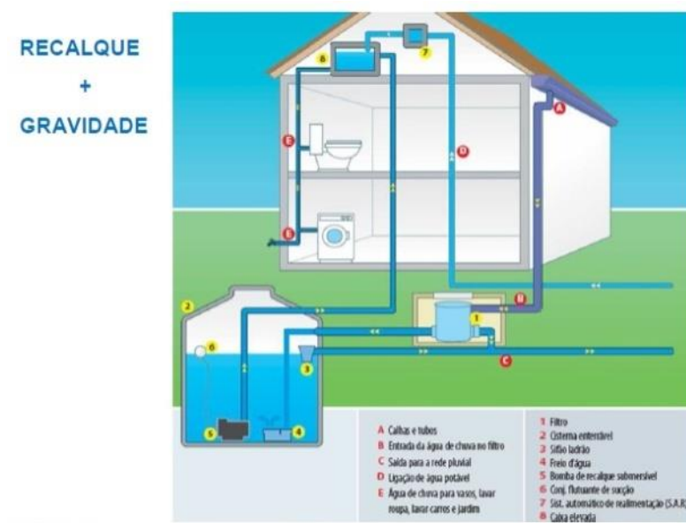
Figura 2 – Sistema Recalque com gravidade. Fonte: Ecoracional 2012
