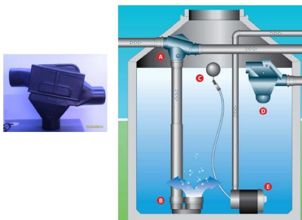
Figura 3 - Esquema cisterna e filtro First Flush. Fonte: Ecoracional 2012
