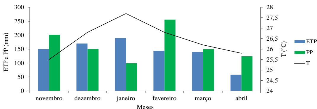
Figura 1. Dados de evapotranspiração potencial (ETP), precipitação pluvial (PP) e temperatura média (T), em Votuporanga, SP, no período estudado, novembro de 2018 a abril de 2019. Fonte: CIIAGRO (2019).
