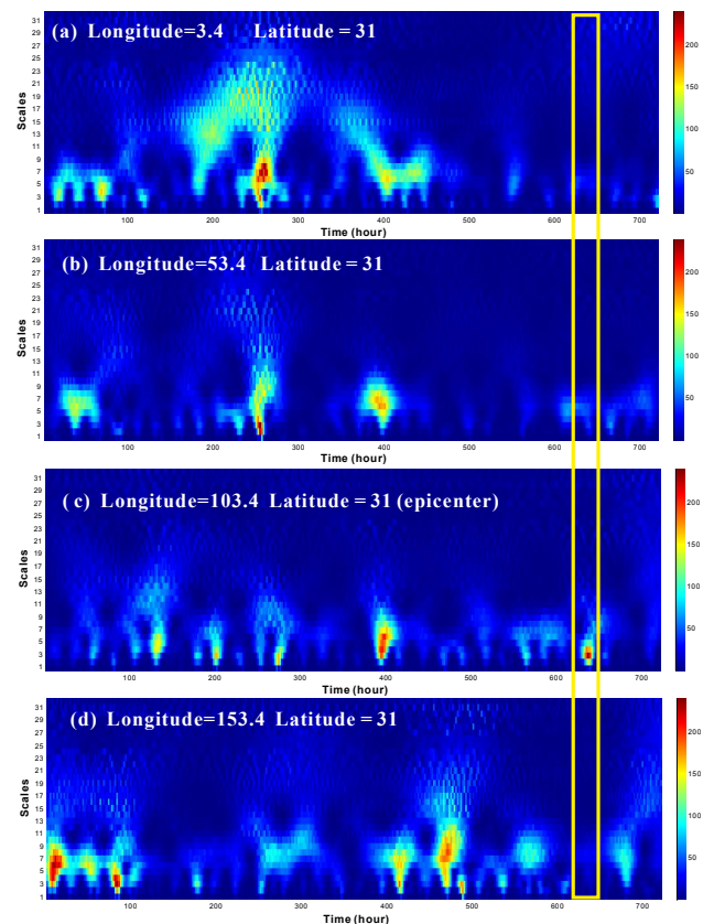
Fig. 3. The analytic wavelet energy density spectrum of DTEC time series from 13 April to 12 May 2008 right over the locations: (a) latitude = 31° N, longitude = 3.4° E; (b) latitude = 31° N, longitude = 53.4° E; (c) latitude = 31° N, longitude = 103.4° E (epicenter); (d) latitude = 31° N, longitude = 153.4° E.
