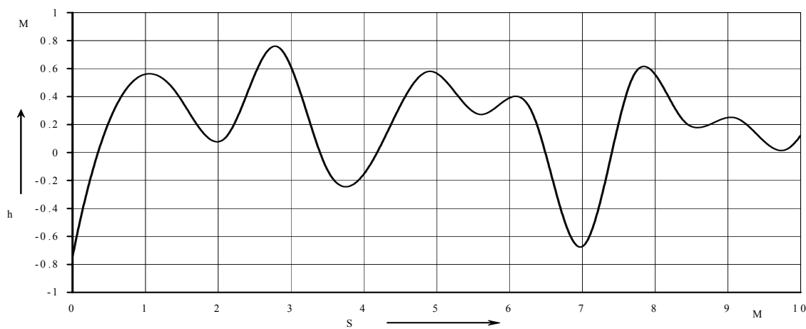
Рис. 6. Результати моделювання мікропрофілю ґрунтової дороги
