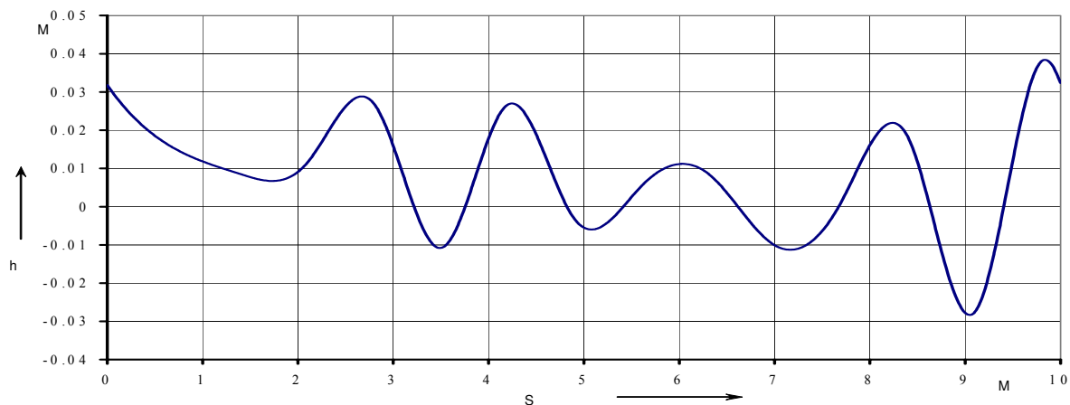
Рис. 5. Результати моделювання мікропрофілю асфальтної дороги
