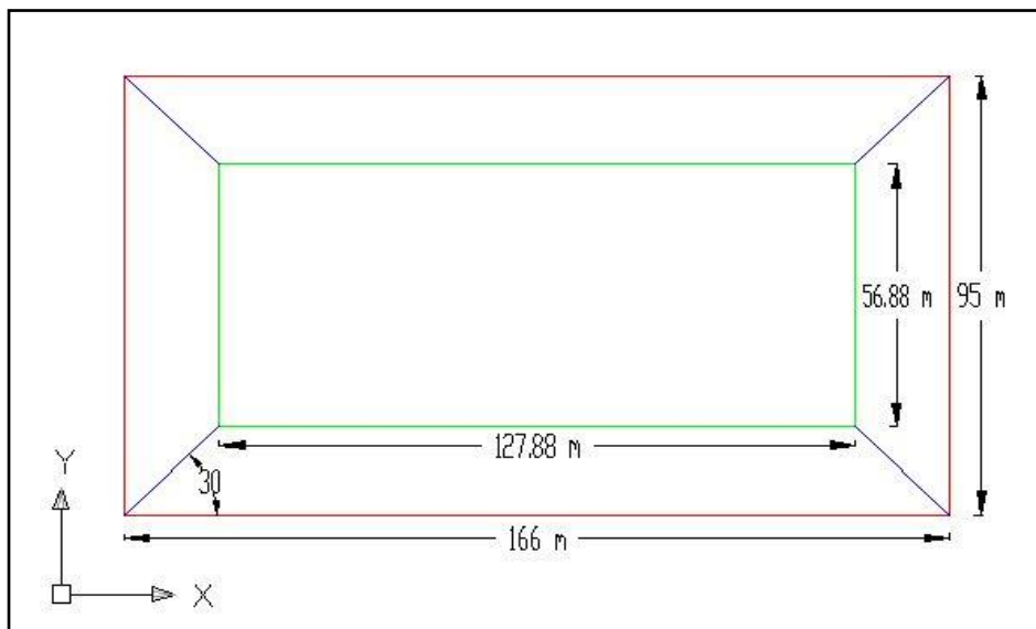
Gambar 14. Desain Layout Perbaikan Area Timbunan 100/200 Tampak Atas
