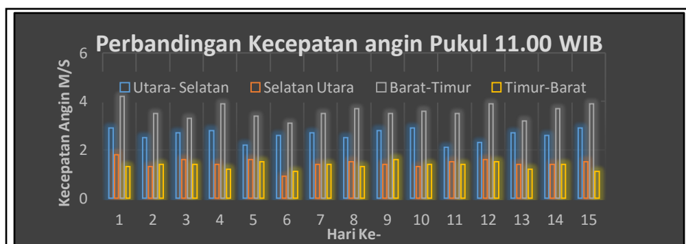
Gambar 8. Perbandingan Kecepatan Angin Pukul 11.00 Wib
