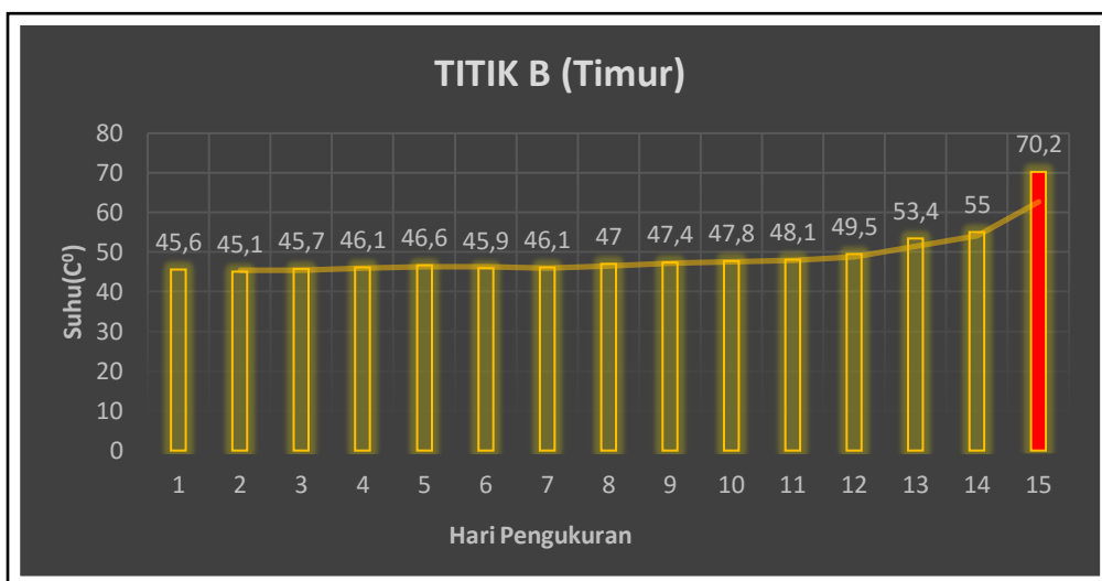
Gambar 3 Grafik Kenaikan Suhu Titik B
