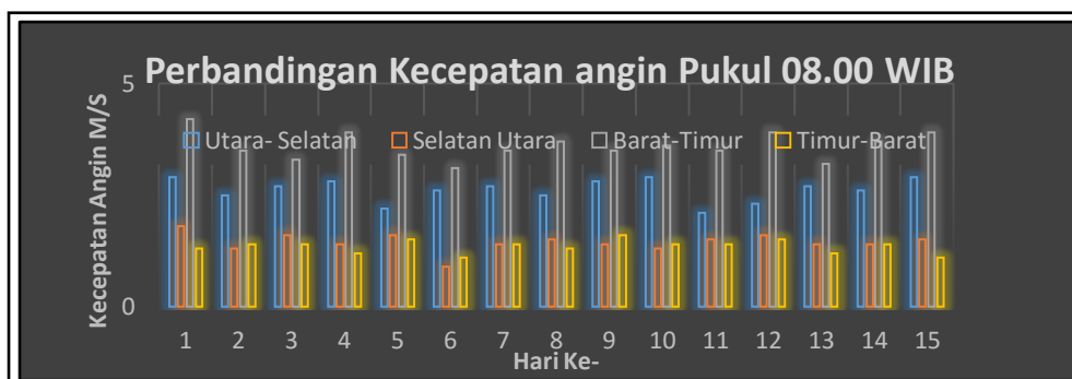
Gambar 7. Perbandingan Kecepatan Angin Pukul 08.00 Wib
