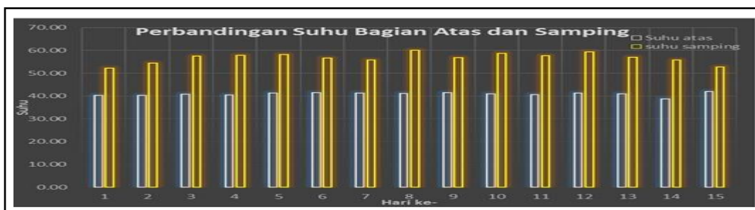
Gambar 6. Perbandingan Suhu Bagian Atas dan Samping Area Timbunan.
