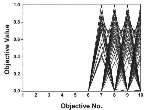
(b) IBEA
