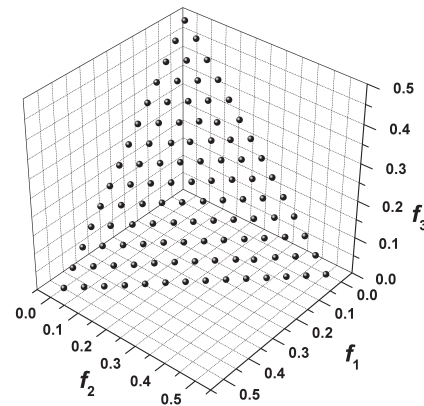
(b) MOEA/D
