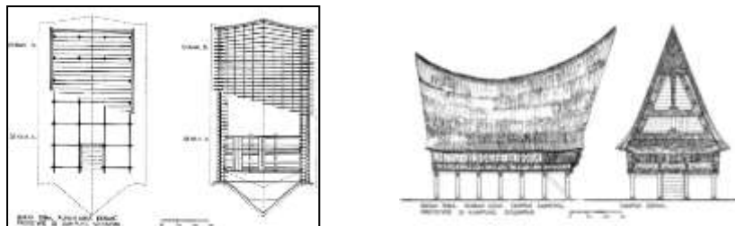
Gambar. 5 Sketsa denah, tampak samping, dan tampak depan Rumah Bolon
