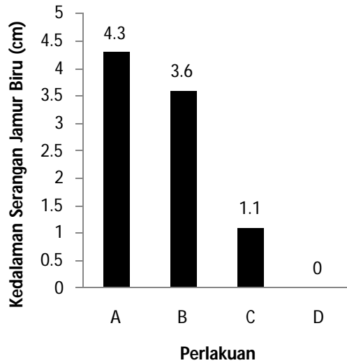
Gambar 6. Kedalaman Serangan Jamur Biru pada Rotan Batang
