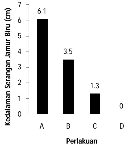
Gambar 7. Kedalaman Serangan Jamur Biru pada Rotan Saloso
