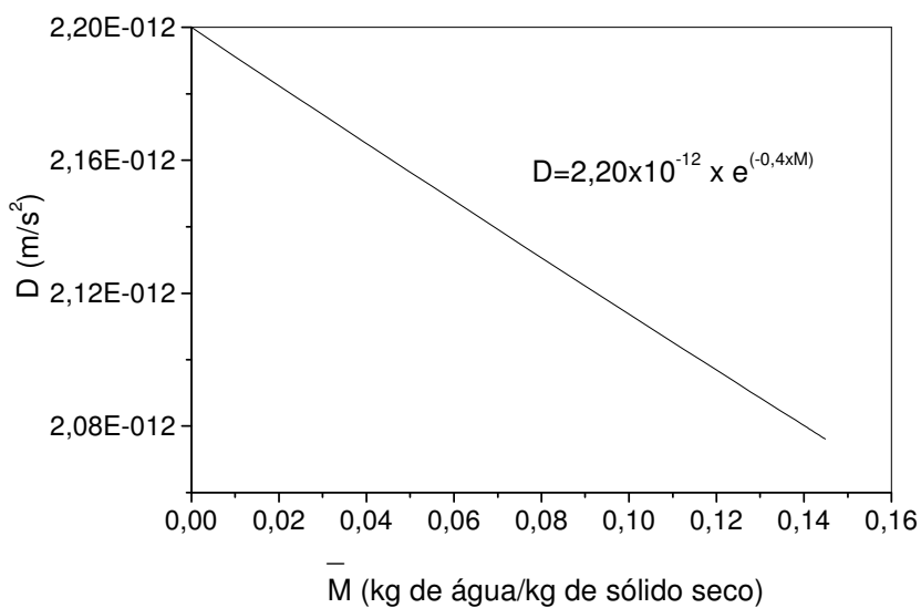
Figura 4.47 - Evolução do coeficiente de difusão em função do teor de umidade médio do compósito reforçado com 30% de fibras, 3mm de espessura e temperatura de 25 °C.
