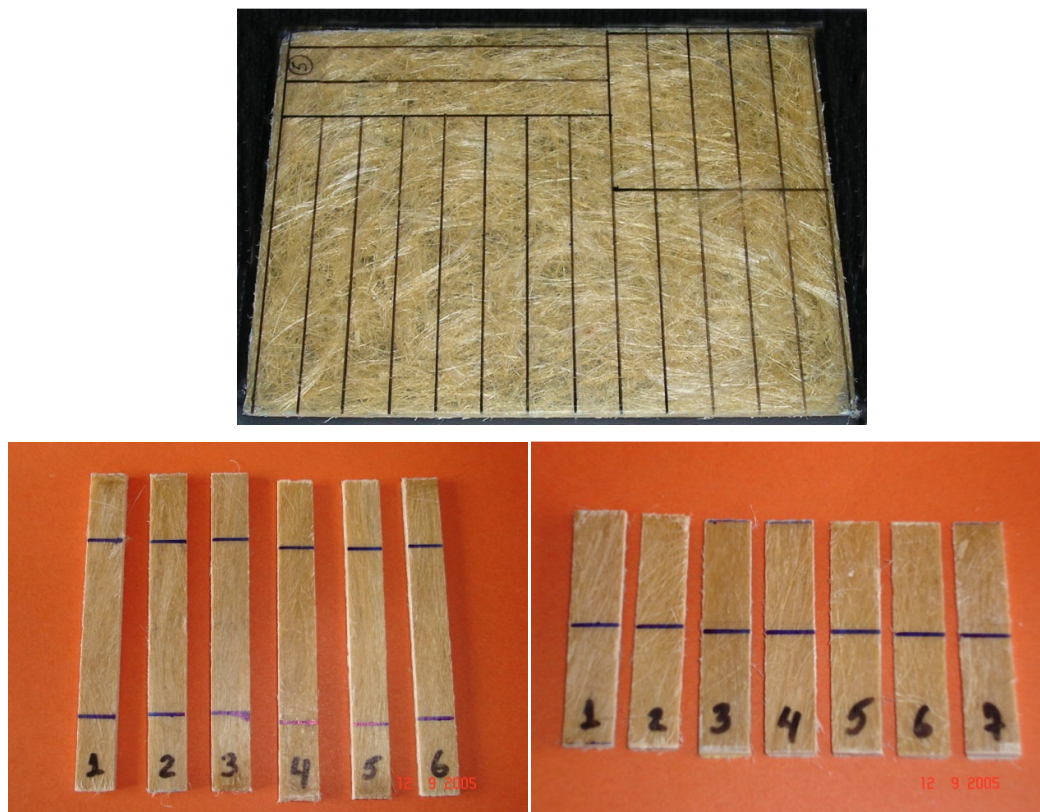
Figura 3.4 – Compósito produzido com fibras de caroá, para ensaios mecânicos.
