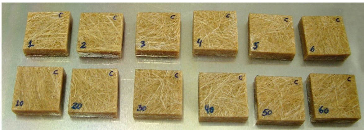
Figura 3.5 – Corpos de prova para ensaio de sorção de água, com 3 e 6 mm de espessura.
