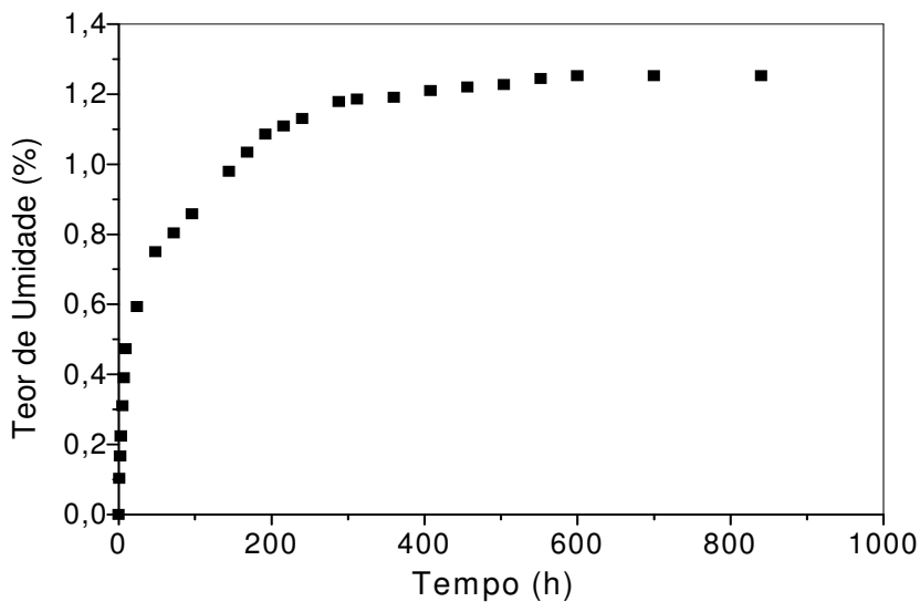
Figura 4.8 - Cinética de sorção de água da resina poliéster insaturado.
