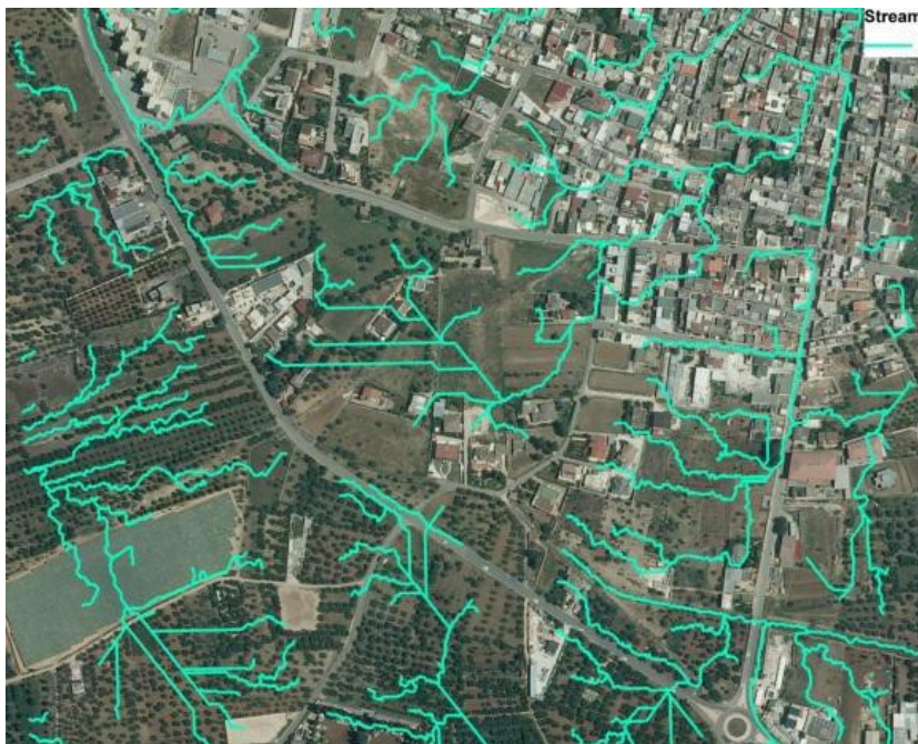
Figura 3b: linee di deflusso superficiale derivate da dato LIDAR.
