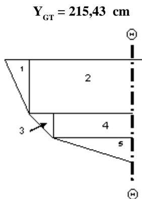
Figura 4. Muestra las cinco áreas de media sección transversal.
