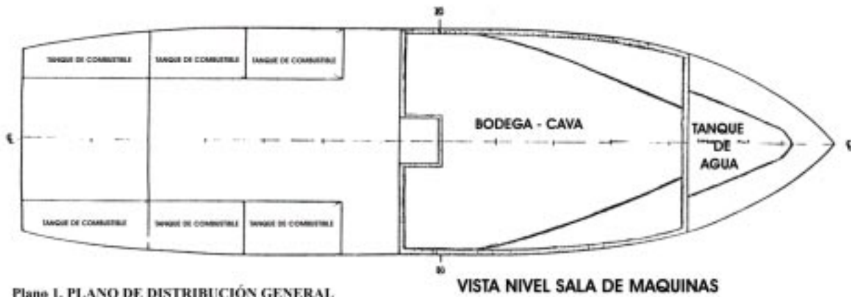
Plano I. PLANO DE DISTRIBUCIÓN GENERAL Diseño y Cálculo: Ing. José Vázquez S. Dibujo: Luis F. González Escala: 1 / 30 Lugar y Fecha: Barcelona, Abril 1989
