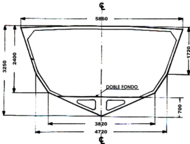
Figura 3. Cuaderna 28, a mitad de la cava.
