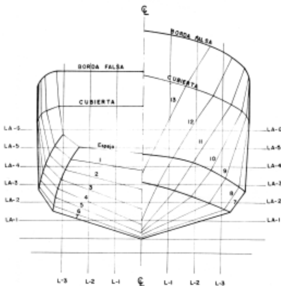
Figura 1. Plano de balizas o caja de cuadernas
