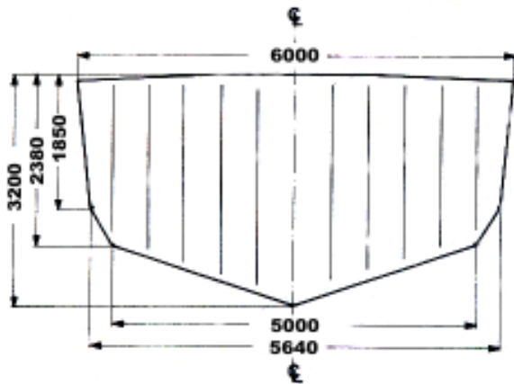
Figura 2. Cuaderna 20, mamparo estanco entre sala de máquinas y cava frigorífica.
