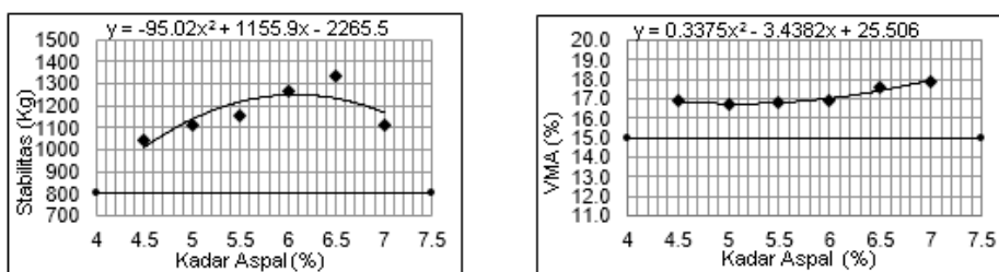
Gambar 3.(a).Grafik Hub.Stabilitas dengan Kadar Laston pada Variasi Kadar Filler 1% (b).Grafik Hub. VMA dengan Kadar Laston pada Variasi Kadar Filler 1%
