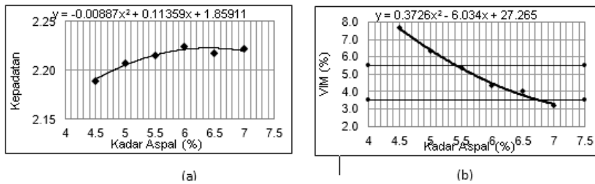
Gambar 2.(a).Grafik Hub.Kepadatan dan Kadar Laston pada Variasi Kadar Filler 1% (b). Grafik Hub.VIM dengan Kadar Laston pada Variasi Kadar Filler 1%
