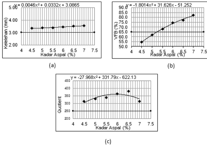
Gambar 4(a). Grafik Hubungan flow dengan Kadar Laston pada Variasi Kadar Filler 1% (b). Grafik Hub. VFB dengan Kadar Laston pada Variasi Kadar Filler 1% (c). Grafik Hub. Quotient dengan Kadar Laston pada Variasi Kadar Filler 1%
