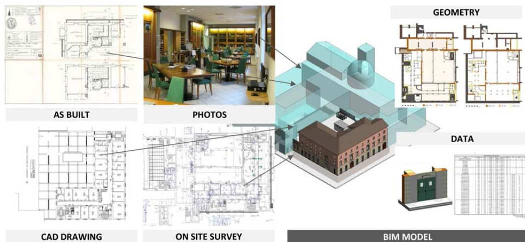
Figure 21: BIM model definition from survey and existing documentation. TOBIM Project. Case study: Archivio Storico della Città di Torino, modelled by Aitana Marcos Guinea.
