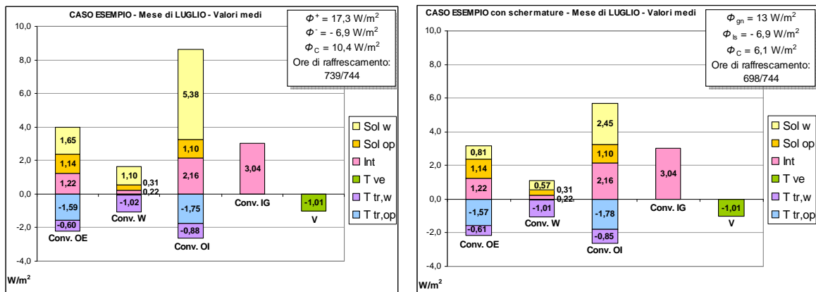
Figura 2.16 Valore medio mensile (luglio) dei termini del bilancio termico in relazione alle sollecitazioni termiche; confronto tra il caso studio nella situazione originaria e con la presenza di schermature solari.
