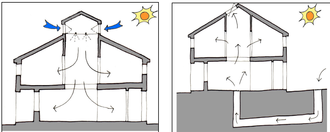
Figura 1.3 Schematizzazione delle strategie di raffreddamento evaporativo, a sinistra, e di raffreddamento geotermico, a destra (fonte: Ford et al. , The Passivhaus Standard in European warm climates. Part 3 , 2007).
