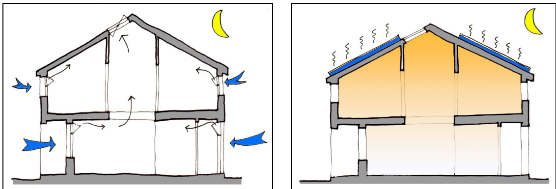
Figura 1.2 Schematizzazione delle strategie di ventilazione notturna, a sinistra, e di raffrescamento radiativo, a destra (fonte: Ford et al., The Passivhaus Standard in European warm climates. Part 3 , 2007).
