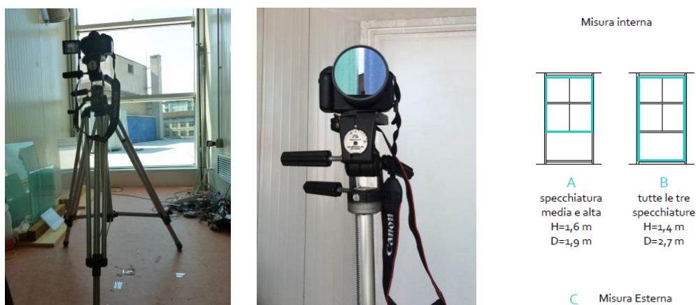
Figura 65 immagini dello strumento di misura e schema delle acquisizioni.
