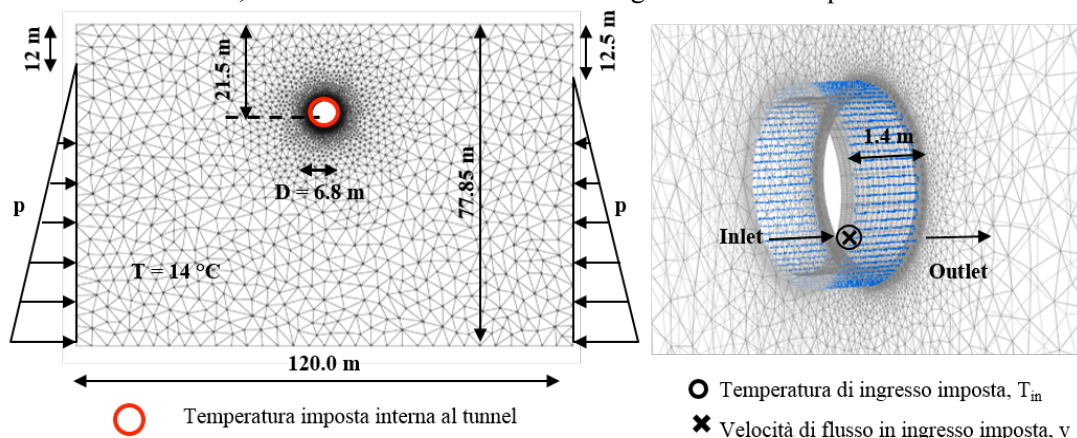
Fig 1. Geometria e dimensioni del modello 3D.
