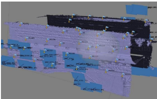
Figura 8 - A sinistra: mesh del fregio elaborata a partire dai dati fotogrammetrici; a destra: mesh del fregio texturizzata con ortofoto estratte dal modello fotogrammetrico.
