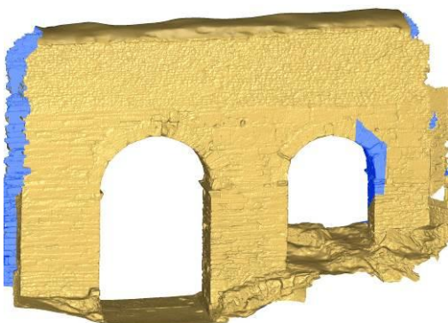
Figura 9 - A sinistra: mesh degli archi dell'acquedotto da dati laser; a destra: mesh del tratto di mura da dati laser texturizzata con dati fotogrammetrici terrestri.
