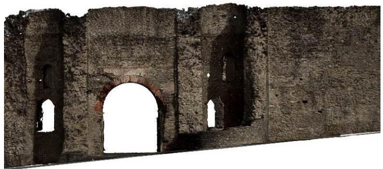
Figura 9 - A sinistra: mesh degli archi dell'acquedotto da dati laser; a destra: mesh del tratto di mura da dati laser texturizzata con dati fotogrammetrici terrestri.
