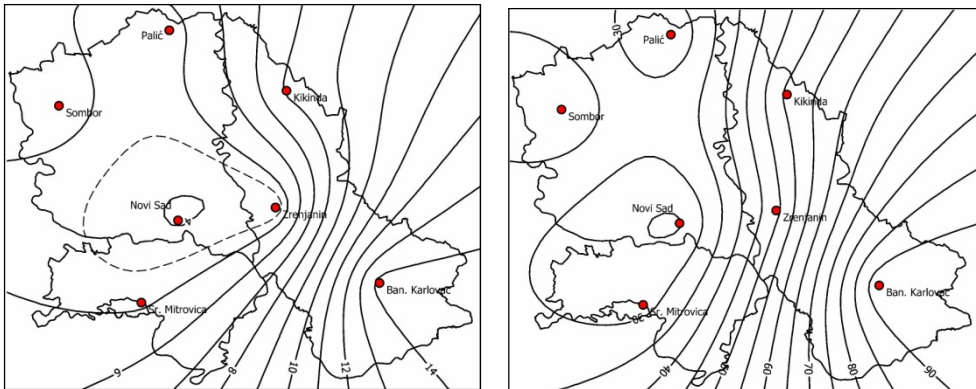
Sl. 2. Izolinije prosečnih i maksimalnih mesečnih vrednosti klimatskog faktora eolske erozije (CF) Isolines of the average and maximum monthly values of the wind erosion climatic factor (CF)
