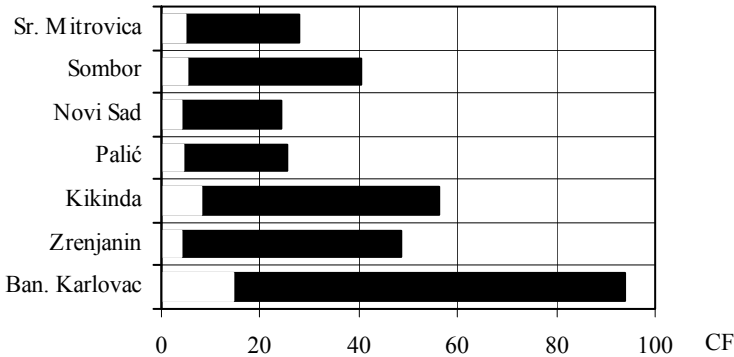
Sl. 1. Raspon od prosečnih do maksimalnih vrednosti klimatskog faktora eolske erozije (CF) za analizirane lokalitete The range from average to maximum values of climatic factors of wind erosion (CF) for analysed localities
