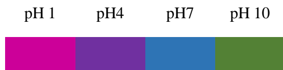
Gambar 03. Warna Antosianin Bunga Telang pada Berbagai pH
