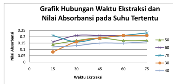
Gambar 04. Grafik Hubungan antara Nilai Absorbansi dengan Waktu Ekstraksi pada berbagai Suhu Ekstraksi (Budiyati et al., 2012)
