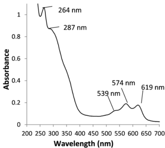
Gambar 02. Nilai Absorbansi Ekstrak Bunga Telang pada pH 4,5 dengan UV-VIS(Marpaung, 2017)
