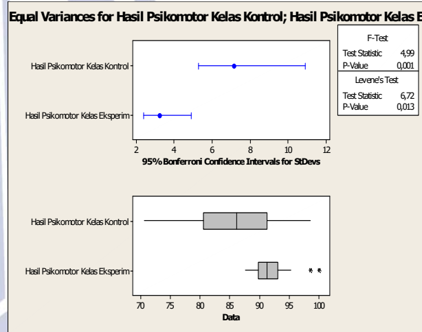
Gambar 23 Uji Homogenitas Psikomotorik 2 variances
