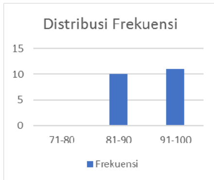
Gambar 17 Distribusi frekuensi rata-rata psikomotor kelas eksperimen
