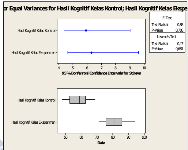
Gambar 22 Uji Homogenitas Kognitif 2 variances
