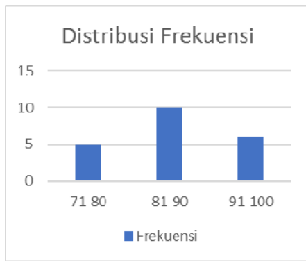
Gambar 16 Distribusi frekuensi rata-rata psikomotor kelas kontrol
