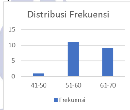
Gambar 14 Distribusi frekuensi rata-rata kognitif siswa kontrol
