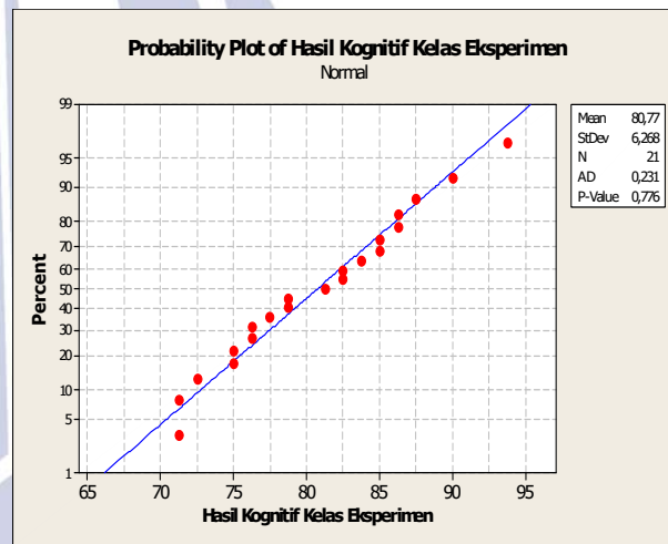
Gambar 19 Uji Normalitas Kognitif Kelas Eksperimen XI TKJ 3
