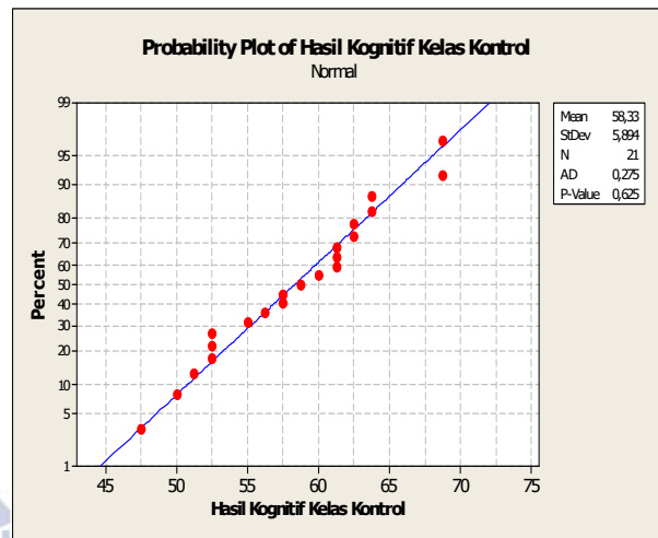
Gambar 18 Uji Normalitas Kognitif Kelas Kontrol X TKJ 3
