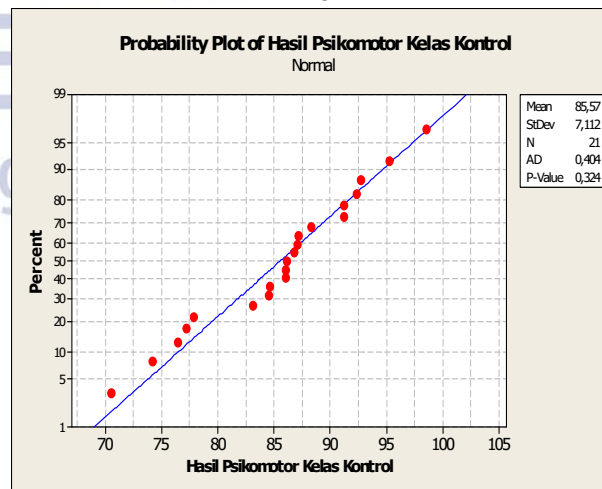
Gambar 20 Uji Normalitas Psikomotorik Kelas Kontrol X TKJ 3
