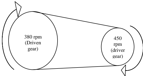
Gambar 3. Rencana Perbandingan Sprocket
