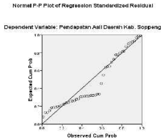
Gambar 4.1 Uji Normalitas
