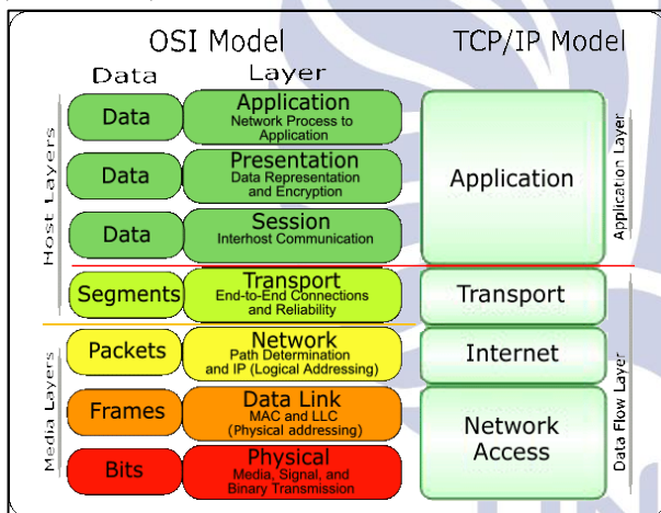
Gambar 1. OSI Layer
