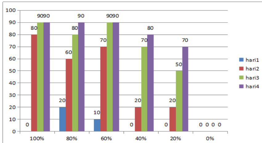
Gambar 1. Diagram batang dinamika mortalitas ulat grayak selama 4 hari perlakuan.
