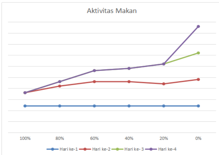
Gambar 2. Data aktivitas makan ulat grayak selama 4 hari pengamatan
