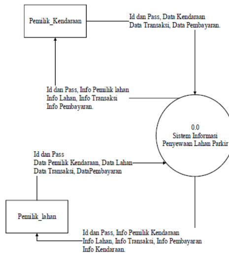
Gambar. 5. Data Flow Diagram Penyewaan Lahan Parkir
