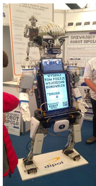
Fot. 7. Robot Dipola 2.0 Fot. S. Bienia.
