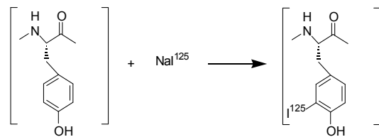
Gambar 1. Skema penandaan ^{125}\text{I} pada polityrosin
