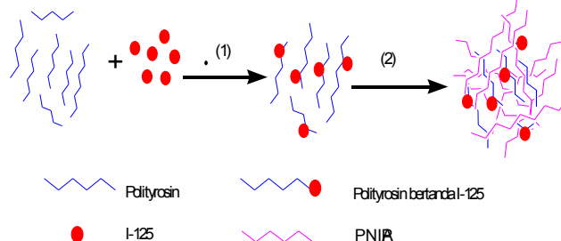
Gambar 2. Skema pembentukan PNIPA/PTYR IPNs bertanda ^{125}\text{I}
