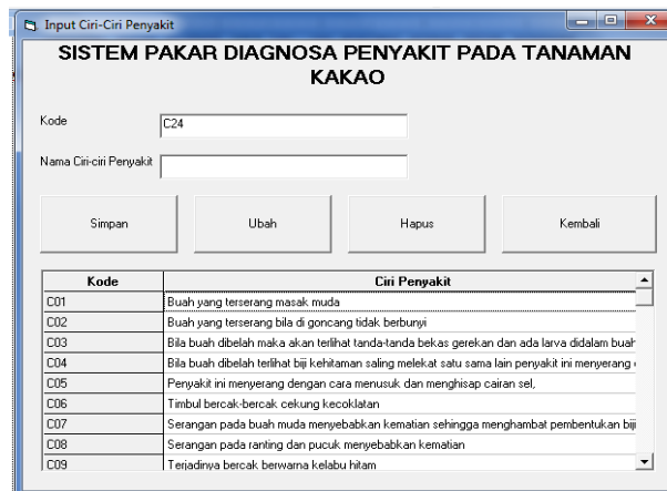
Gambar 9 Input Ciri
