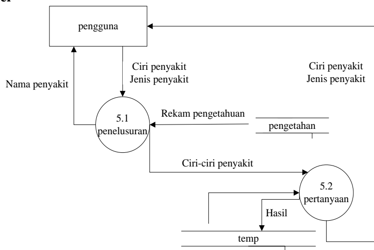
Gambar 5 DFD Level
