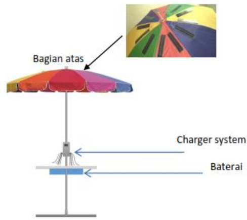
Gambar 5 Design payung charger Sumber : Hasil data primer
