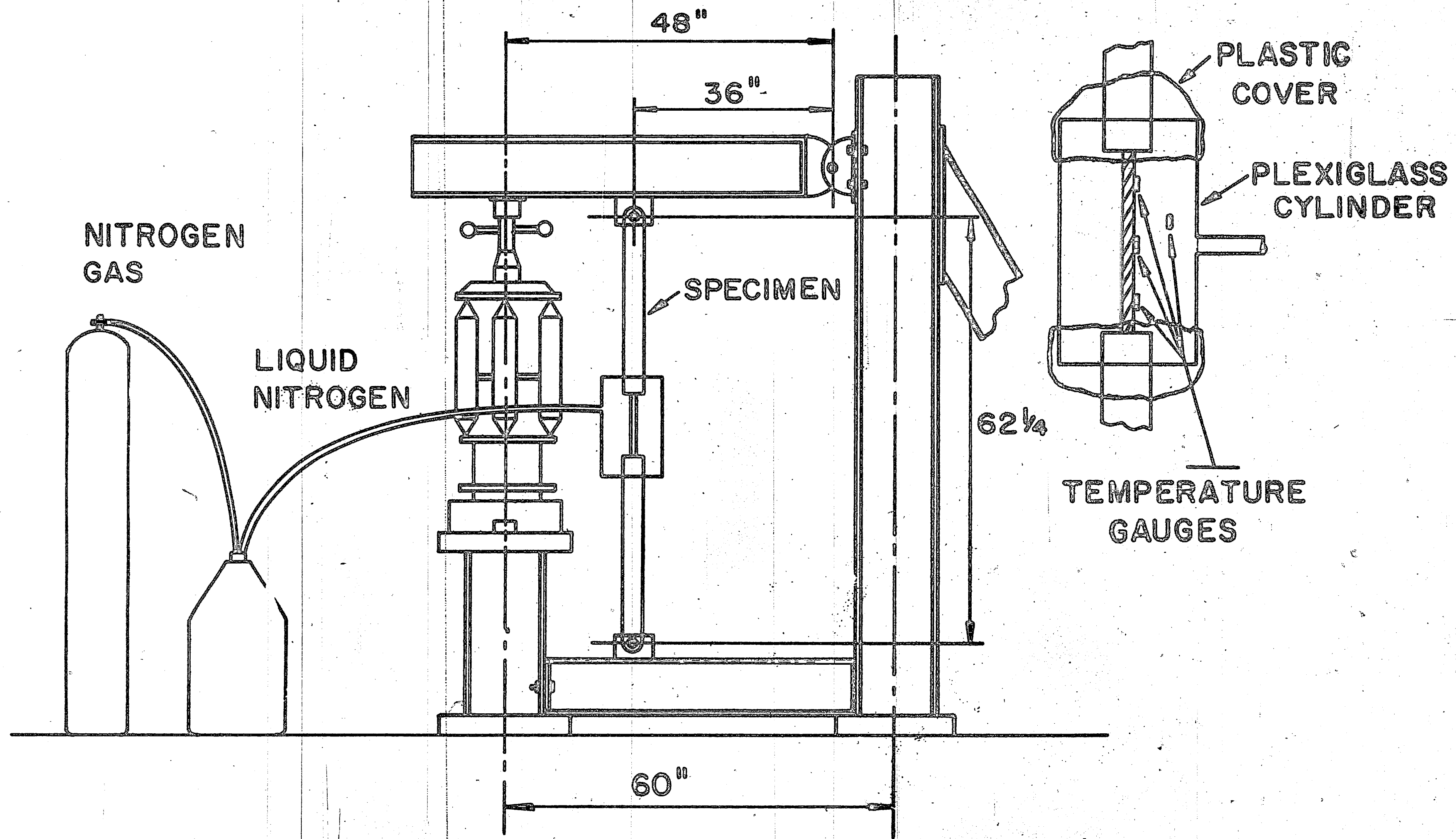
Fig. 10 Fatigue Test Setup
