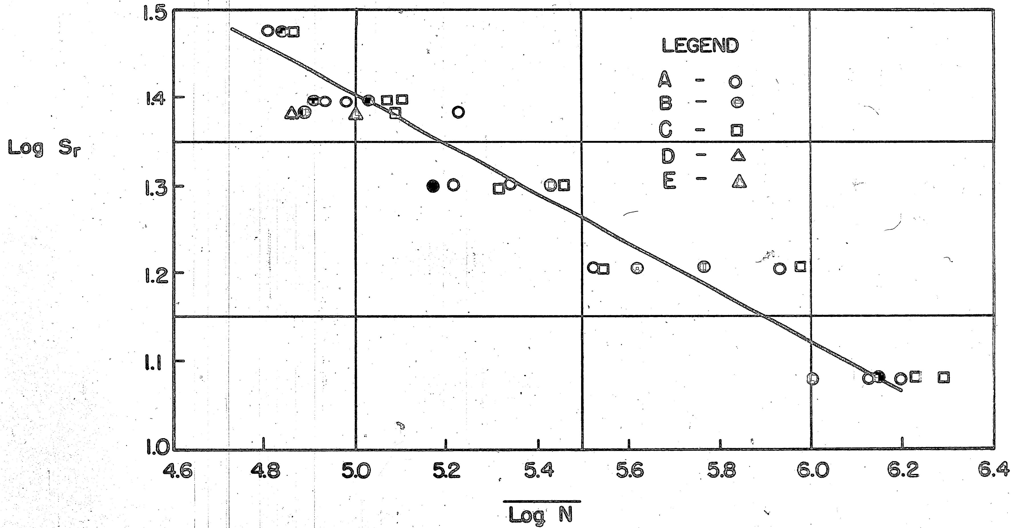
Fig. 23 \overline{\text{Log N}} vs. \text{Log } S_r
