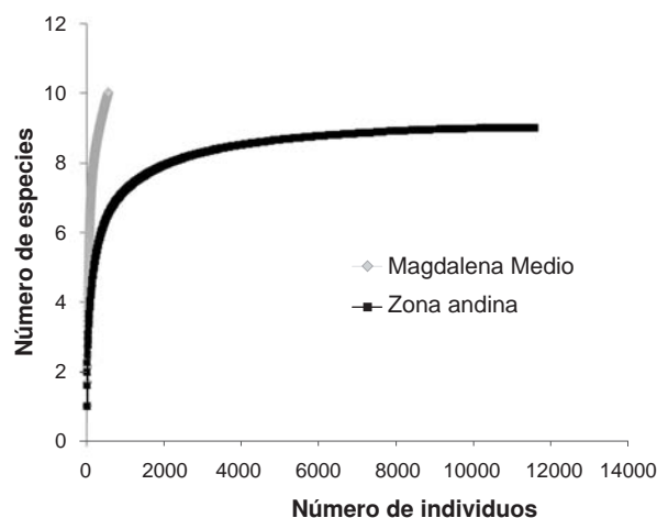
Figura 2. Curvas de acumulación de las especies de triatominos en Santander. A: Zona andina. B: Magdalena Medio. ( \pm CI 95% ). Se utilizó el número de individuos registrados entre 1996 y 2008.
