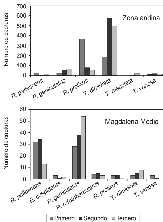
Figura 4. Variación temporal o persistencia de triatominos. Se ilustra la presencia de las especies de triatominos más abundantes en tres períodos, con número de capturas similares en dos regiones del departamento.
