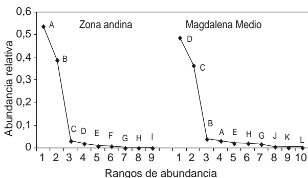
Figura 3. Curvas de rango y abundancia de triatominos en dos zonas del departamento de Santander
