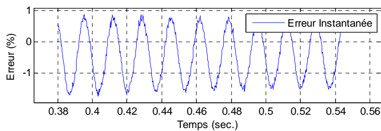
Figure F.5 : Essai No 2 symétrique - SAMU No 3
