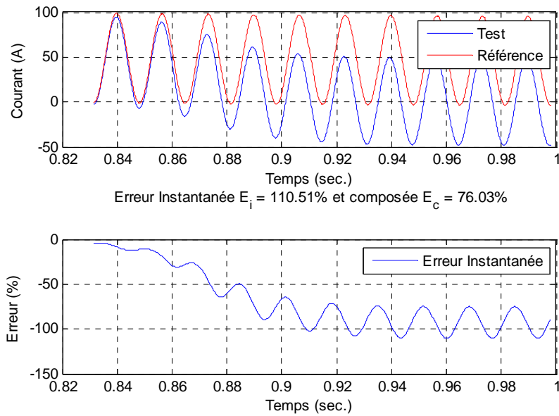
Figure E.3 : Essai No 3 asymétrique - SAMU No 2
