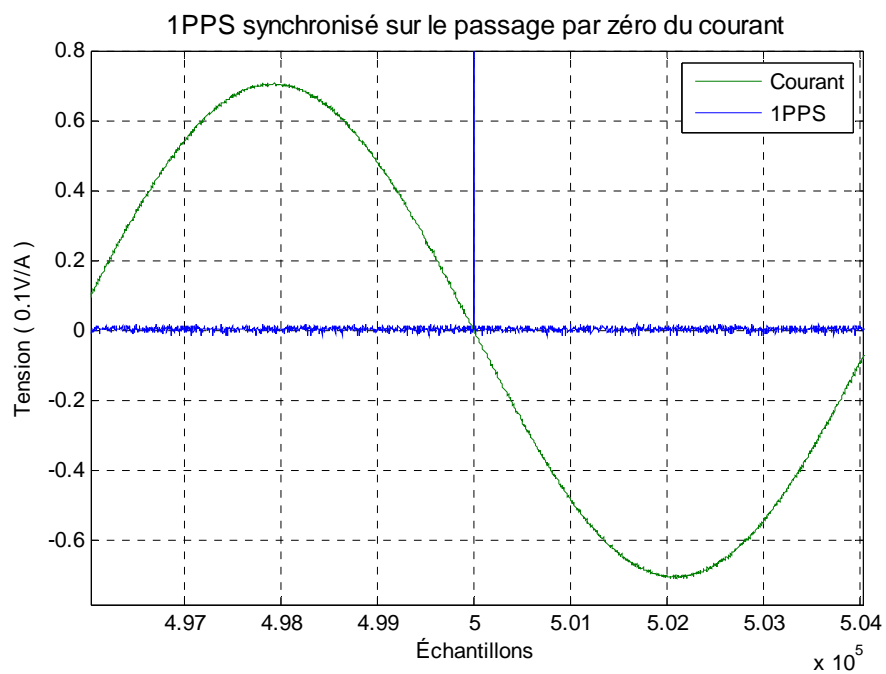
Figure 8.2 : Synchronisation sur le passage par zéro et l'impulsion à 1PPS
