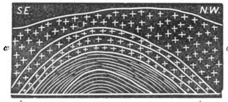
FIG. 2.—Anticlinal N.E. of Pentre'r felin.
