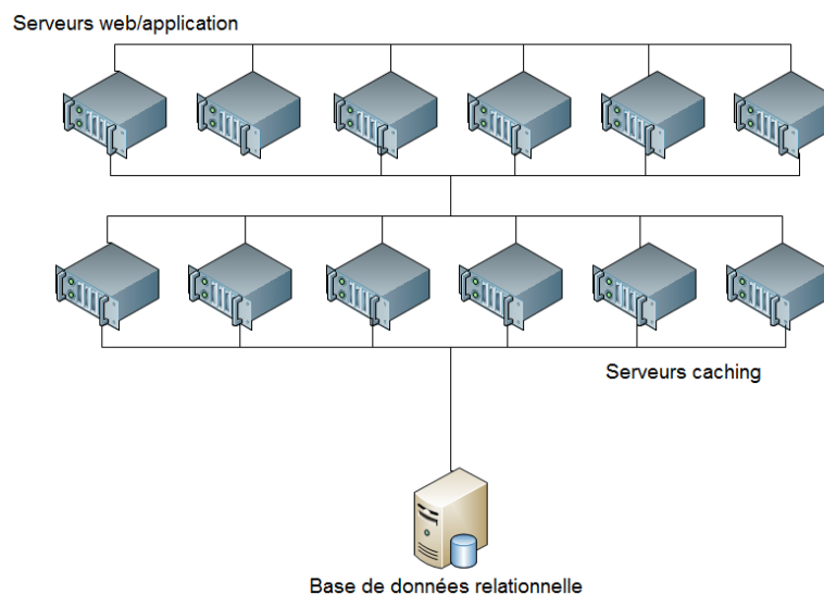
Figure 17 – «Caching» distribué
