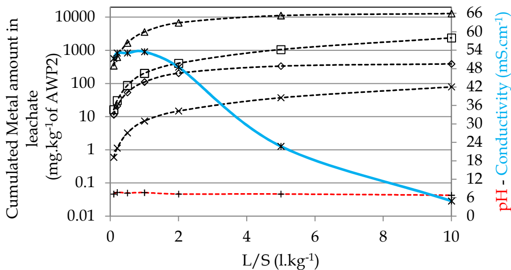
Figure 93 : Percolated amount of calcium (--□--), phosphorus (--◇--), sulfur (--Δ--) and strontium (--×--) from column percolation test of AWP2 blend in function of leaching time, pH (--+--) and conductivity (—+—)
