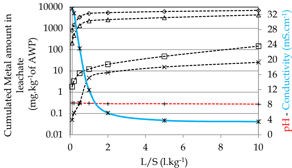
Figure 90 : Percolated amount of calcium (---□---), phosphorus (---◇---), sulfur (---Δ---) and strontium (---×---) from column percolation test of AWP blend in function of leaching time, pH (---+---) and conductivity (---*---)
