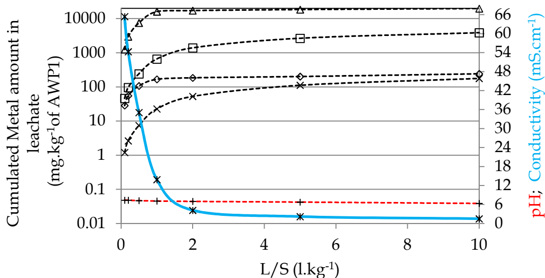
Figure 92 : Percolated amount of calcium (--□--), phosphorus (--◇--), sulfur (--Δ--) and strontium (--×--) from column percolation test of AWP1 blend in function of leaching time, pH (--+--) and conductivity (—+—)
