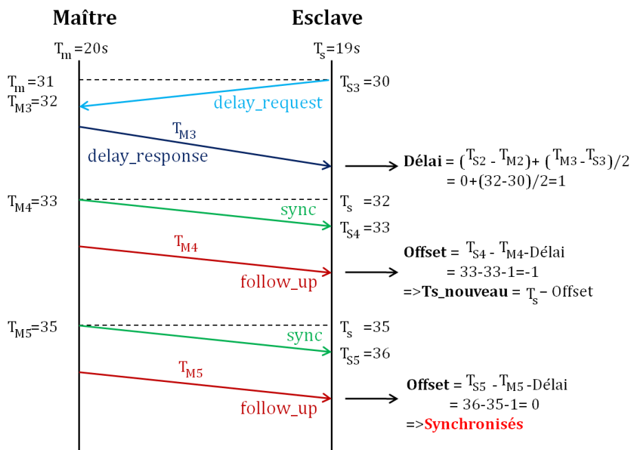
Figure III.2 La deuxième phase de synchronisation de l'IEEE-1588.
