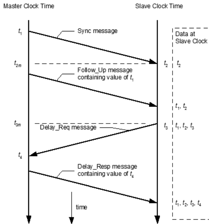
Figure V.10 Fonctionnement d'IEEE-1588 40 .
