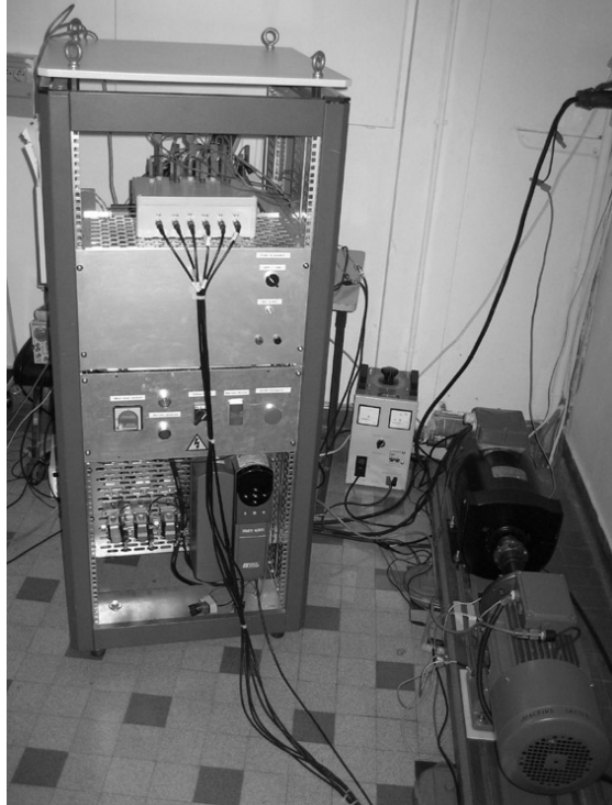
FIG. A.1 – Photographie du banc de test
