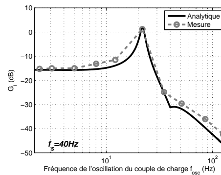
(d) f_s = 40 \text{ Hz}
