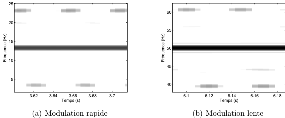
FIG. 6.26 – Zoom sur les DWV de courants statoriques en présence d'oscillations du couple de charge, obtenues à partir du vecteur de Concordia
