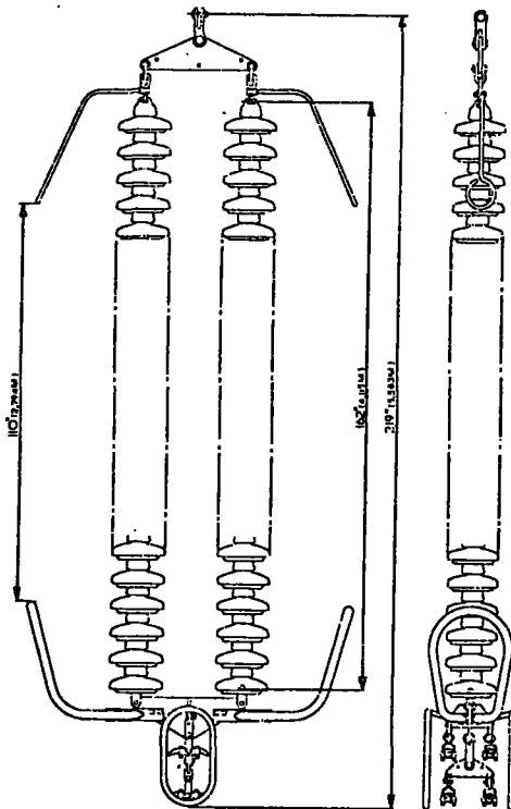
400 kV (quad)
